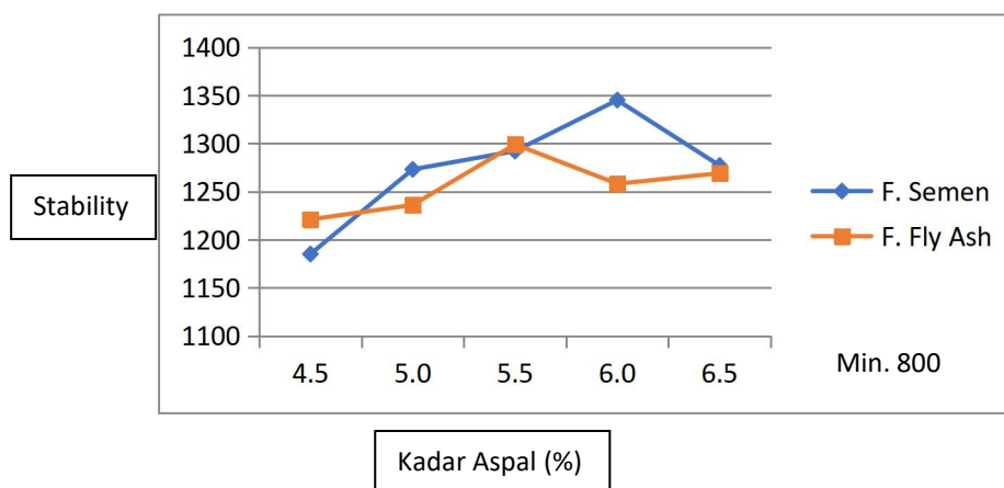
Gambar 5: Grafik Hubungan antara Kadar aspal dan Stability
