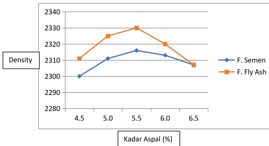
Gambar 1: Grafik Hubungan antara Kadar aspal dan Kepadatan
