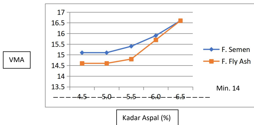
Gambar 2: Grafik Hubungan antara Kadar Aspal dan VMA
