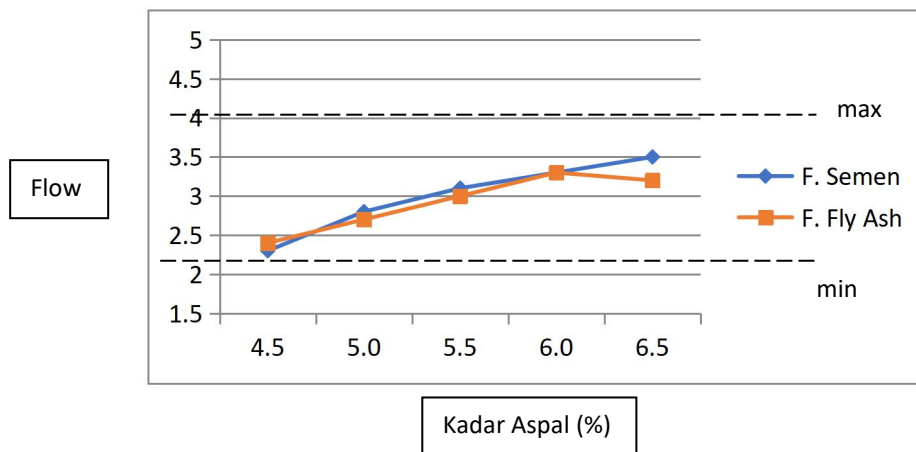
Gambar 6: Grafik Hubungan antara Kadar aspal dan Flow
