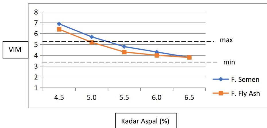
Gambar 4: Grafik Hubungan antara Kadar aspal dan Void in Mix
