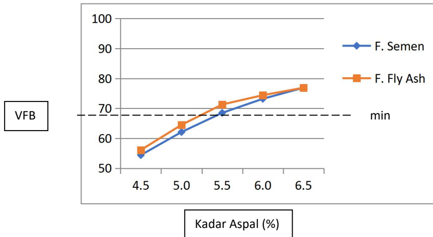
Gambar 3: Grafik Hubungan antara Kadar Aspal dan VFB
