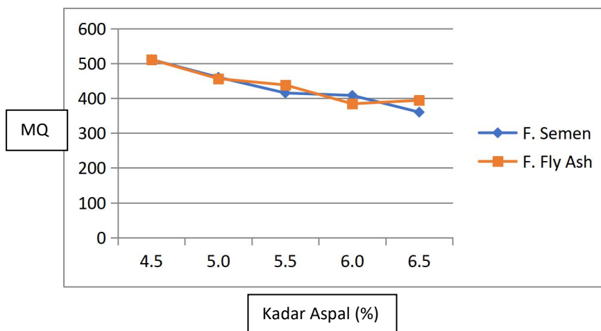
Gambar 7: Grafik Hubungan antara Kadar aspal dan MQ
